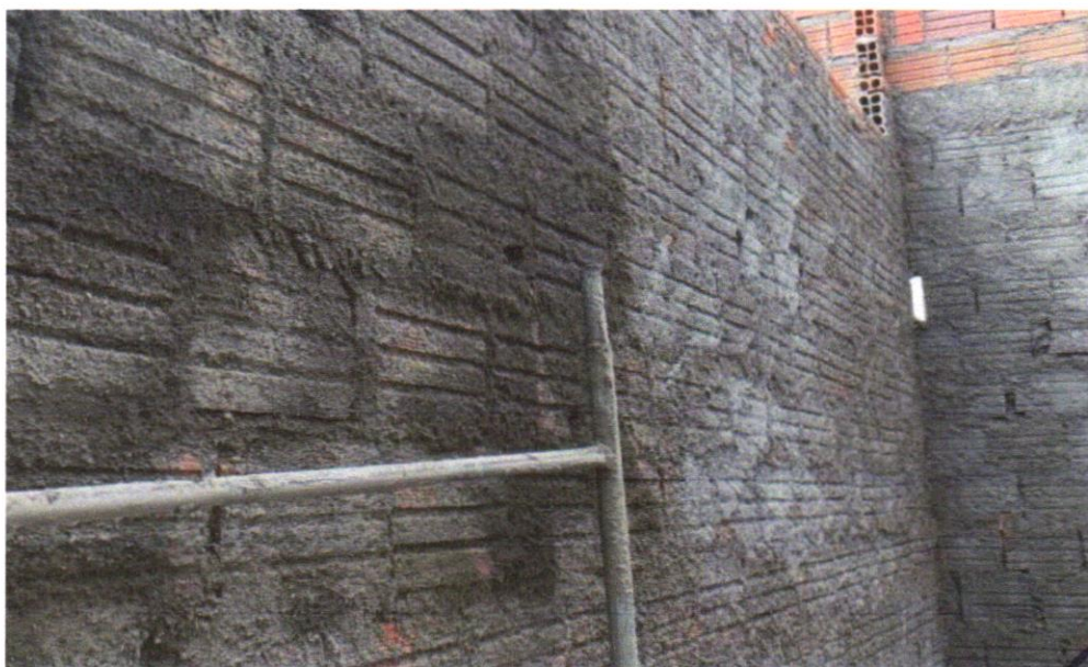
FOTO 08 - CHAPISCO APLICADO EM ALVENARIAS E ESTRUTURAS DE CONCRETO INTERNAS, COM COLHER DE PEDREIRO. ARGAMASSA TRAÇO 1:3 COM PREPARO EM BETONEIRA 400L. AF_06/2014
